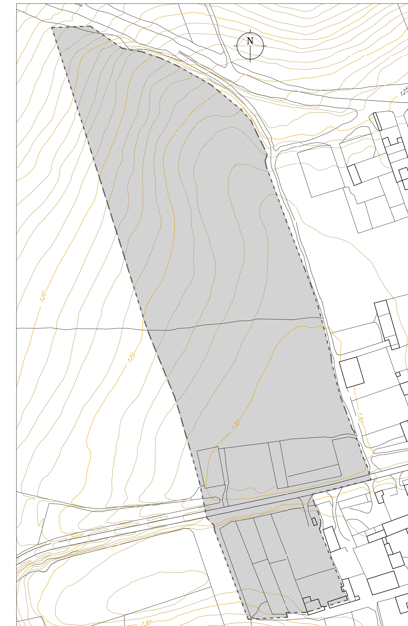
EMPLAZAMIENTO. ESCALA 1/2000.
